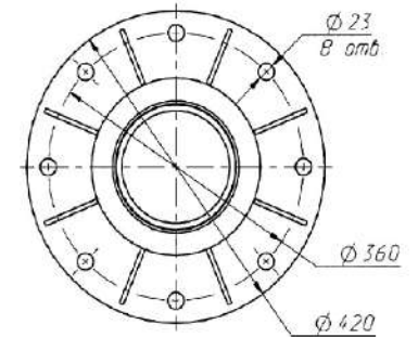
Вид сверху (1.5)
